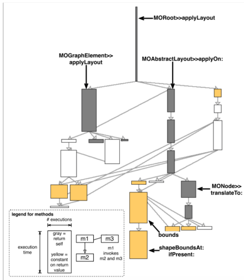
Figura 51: Exemplo da visualização comportamental proposta por Bergel, Robbes e Binder[26].
