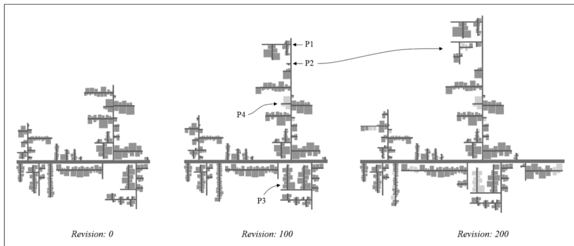
Figura 3: CrocoCosmos [54].
