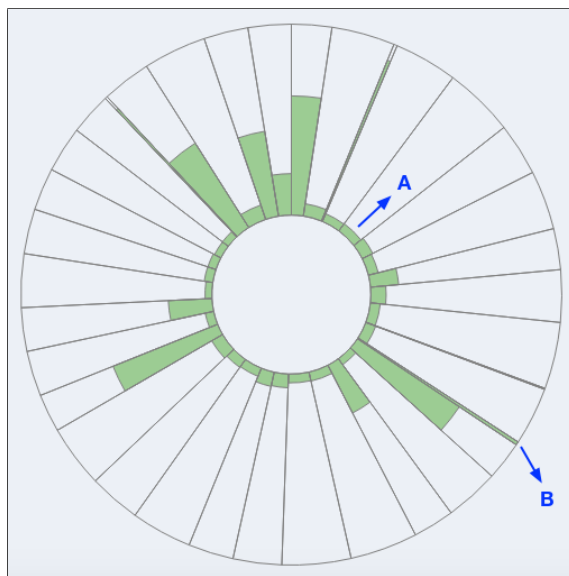
(a) Jetty, 9.3.11/9.3.12.
