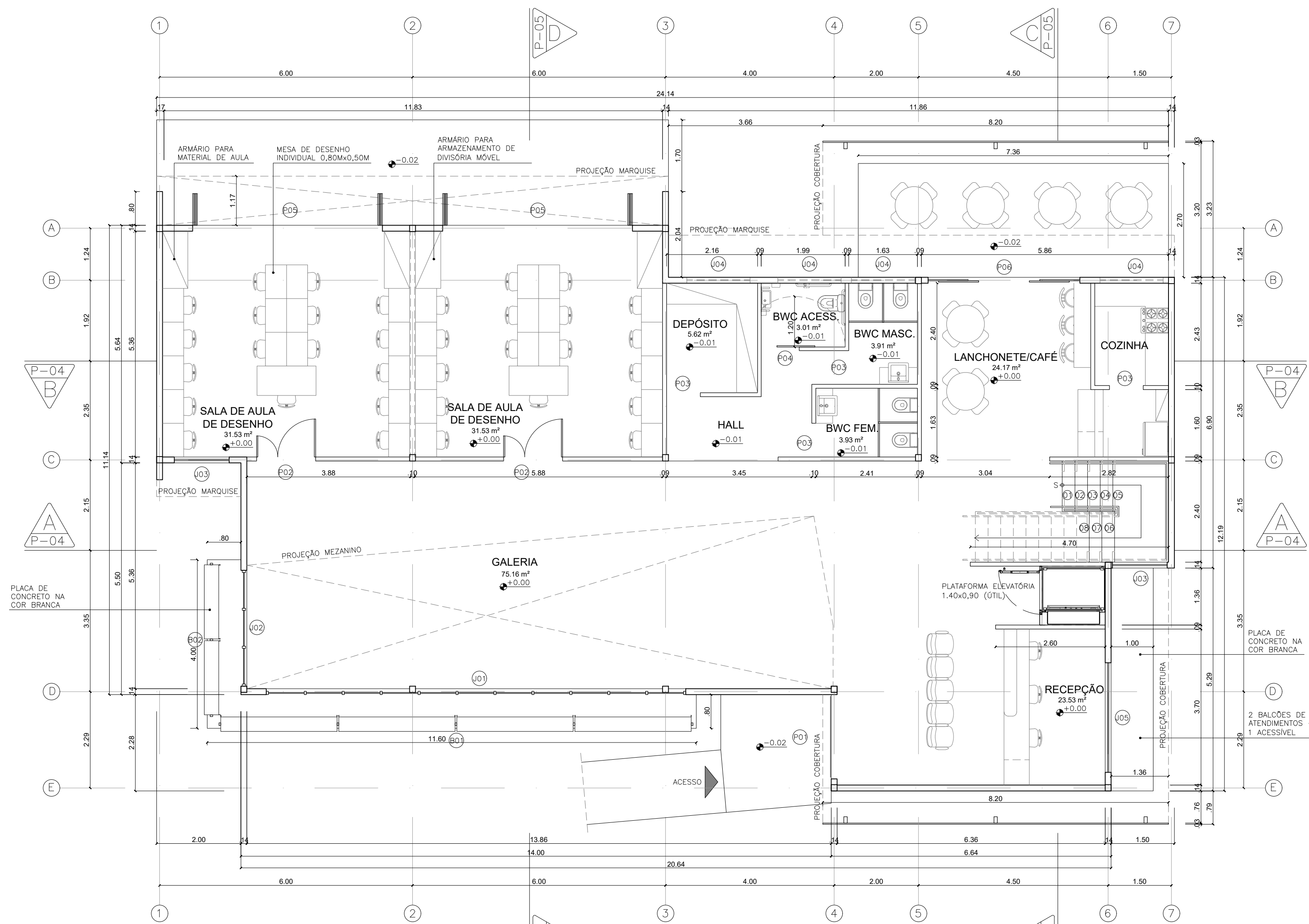
PLANTA BAIXA PAV. TÉRREO ESC. 1/75 253.76 m 2
