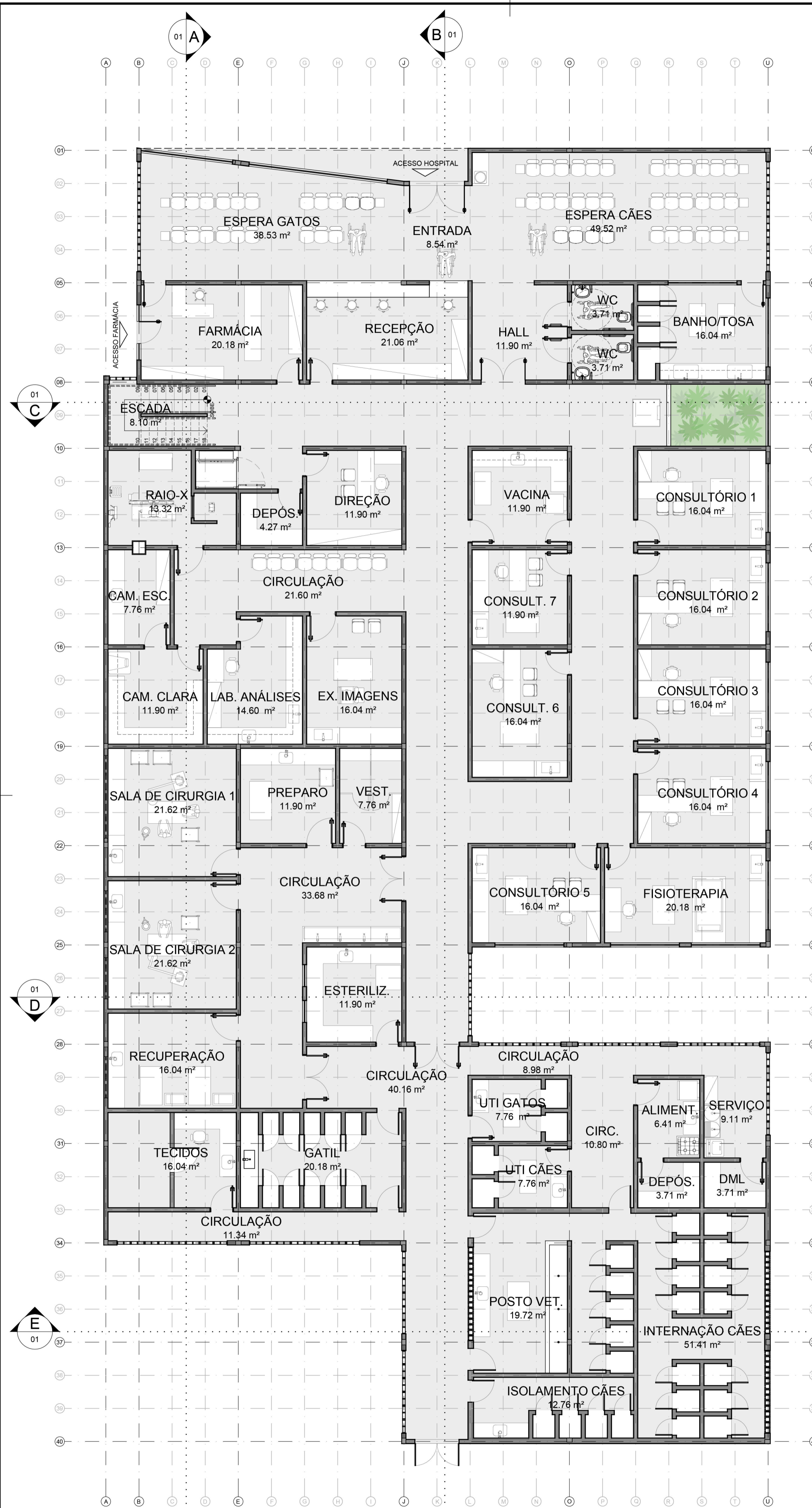
PLANTA DE LAYOUT PAV. TÉRREO ESCALA 1/100
