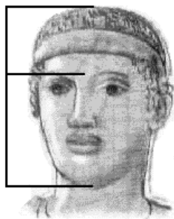
Figura 4.17: Padrão de Harmonia
