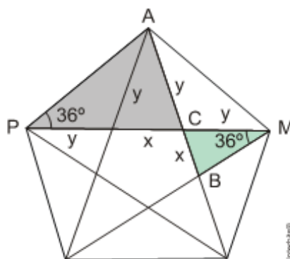
Figura 4.12: Pentágono e triângulos semelhantes
