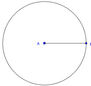
Figura 4.2: Circunferência \alpha
