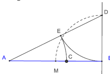
Figura 4.6: Média e extrema razão
