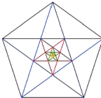
Figura 3.4: Sequência infinita de pentágonos regulares e pentagramas
