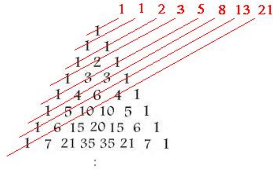
Figura 1.11: Triângulo de Pascal e a sequência de Fibonacci
