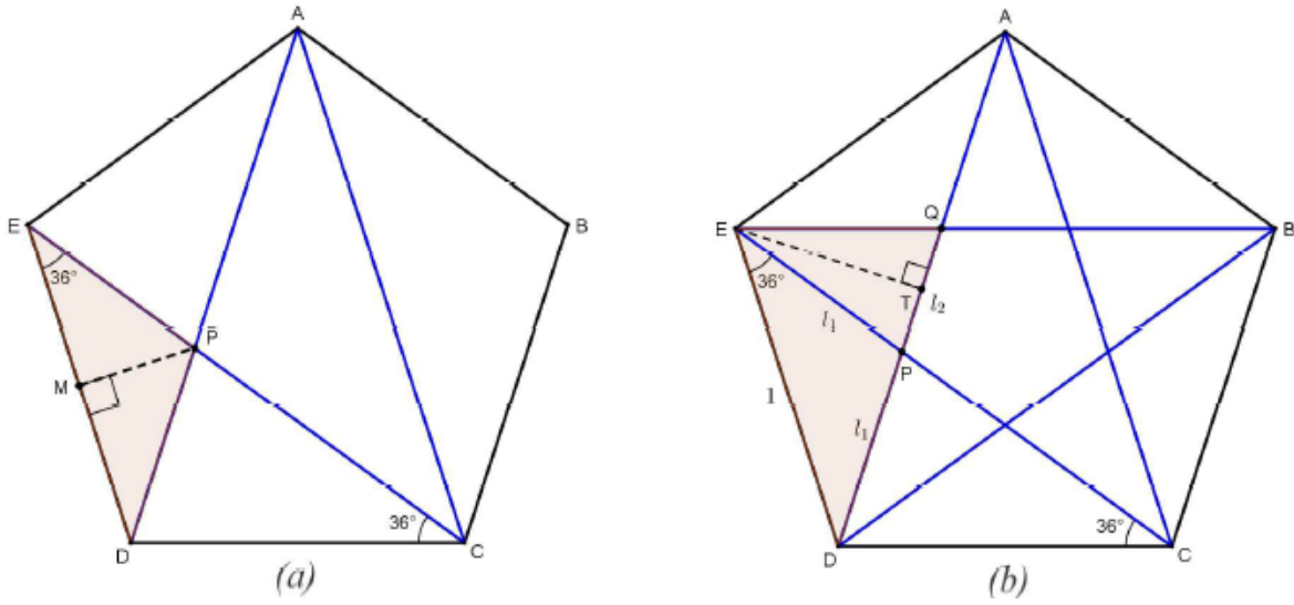
Figura 3.5: Triângulos no pentágono
