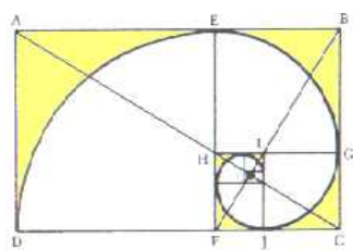
Figura 1.6: Diagonais da espiral
