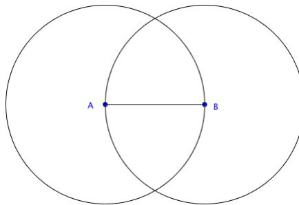
Figura 4.3: Circunferência \beta
