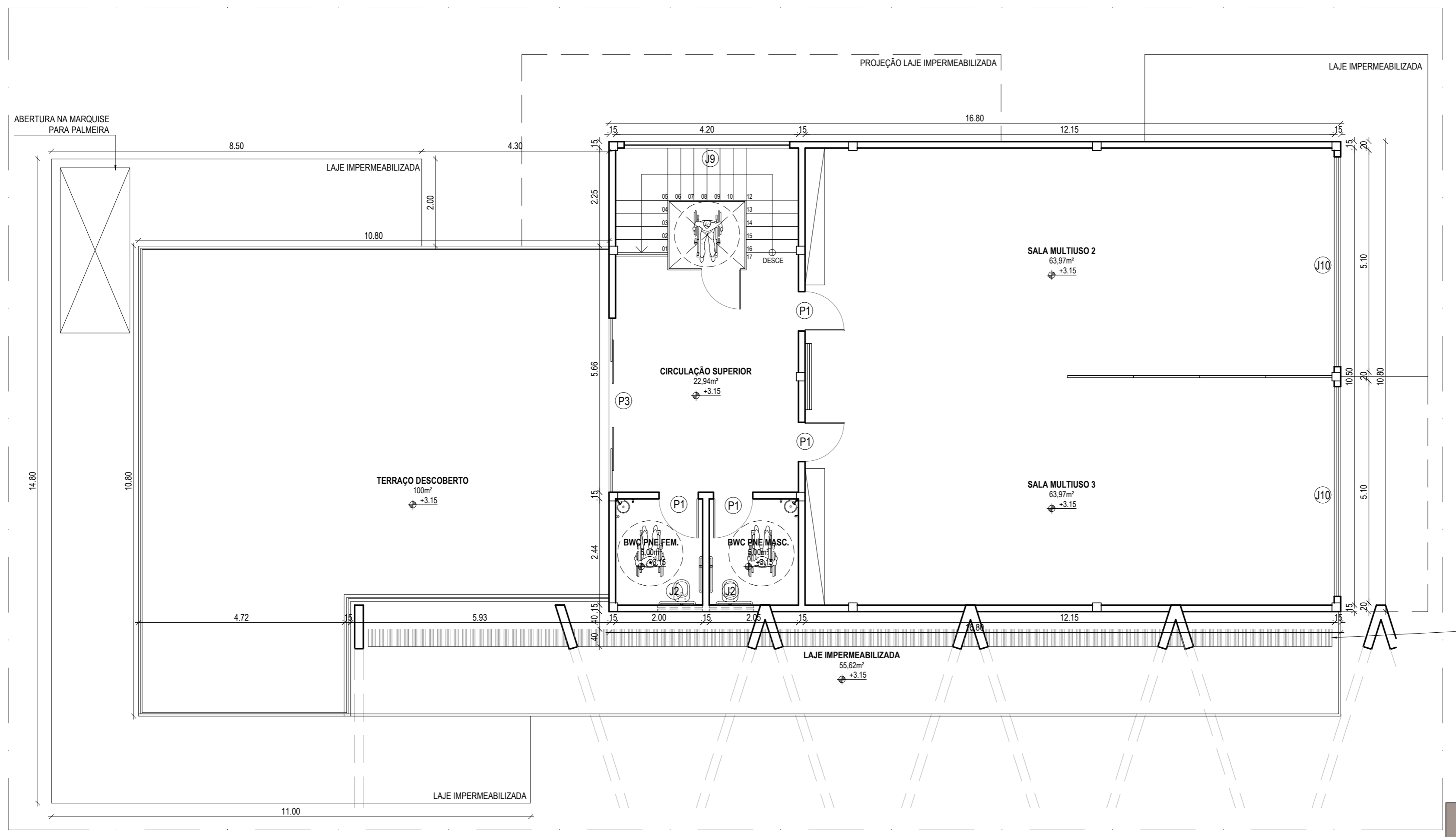
PLANTA BAIXA - 1º PAV. escala 1:75
